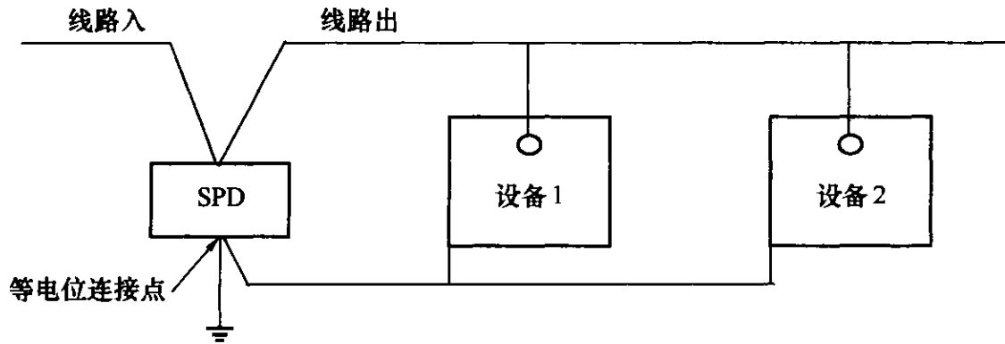
图 11 凯文接线法
