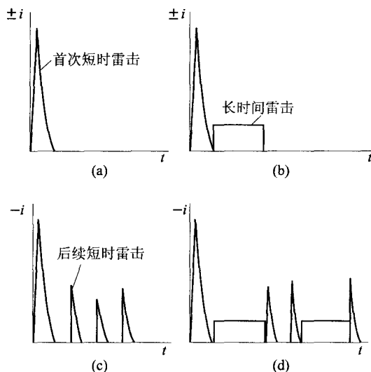
图 21 向下闪击可能的雷击组合
