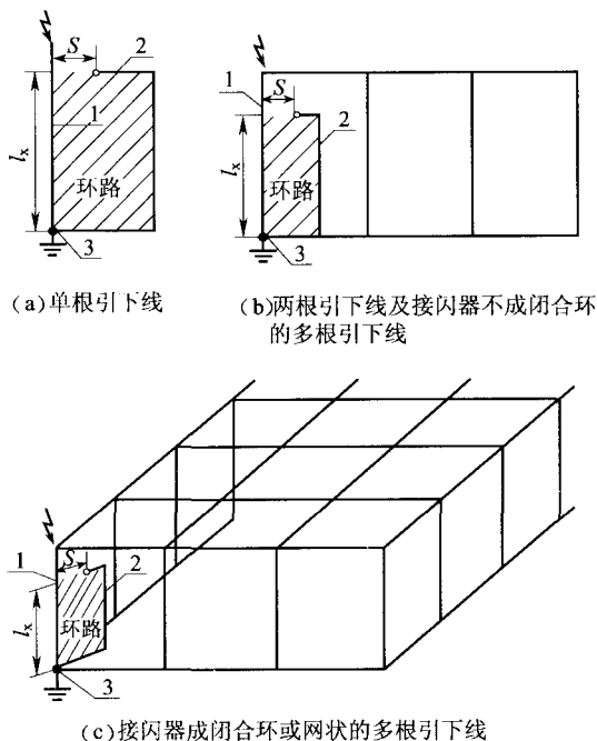
图 E.0.1 分流系数 k_c(1)
