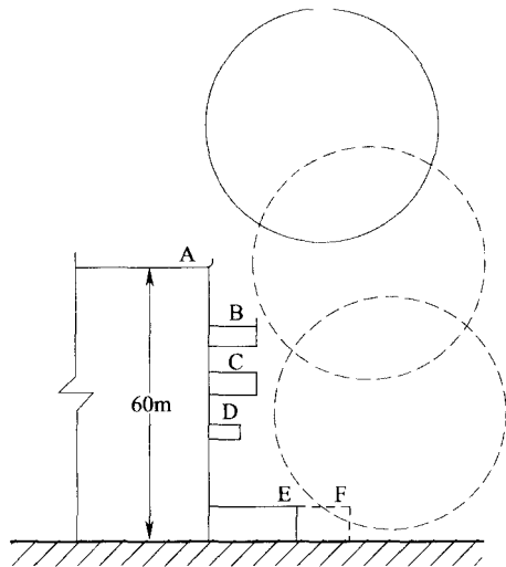
图 14 剖面示意
