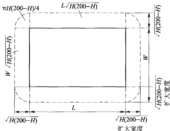
图 A.0.3 建筑物的等效面积
