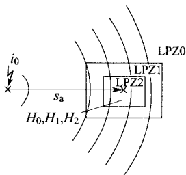
图 6.3.2-1 附近雷击时的环境情况
