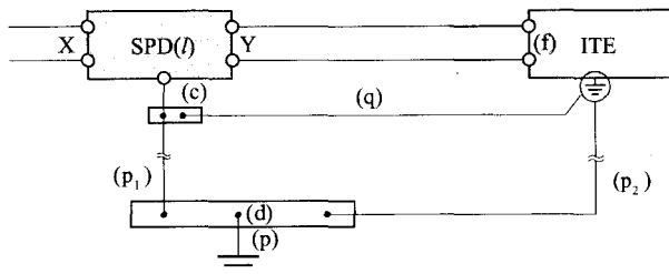
图 J.2.3-2 将多接线端子电涌保护器的有效电压保护水平减至最小所必需的
