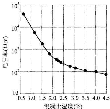
图 12 混凝土湿度对其电阻率的影响
